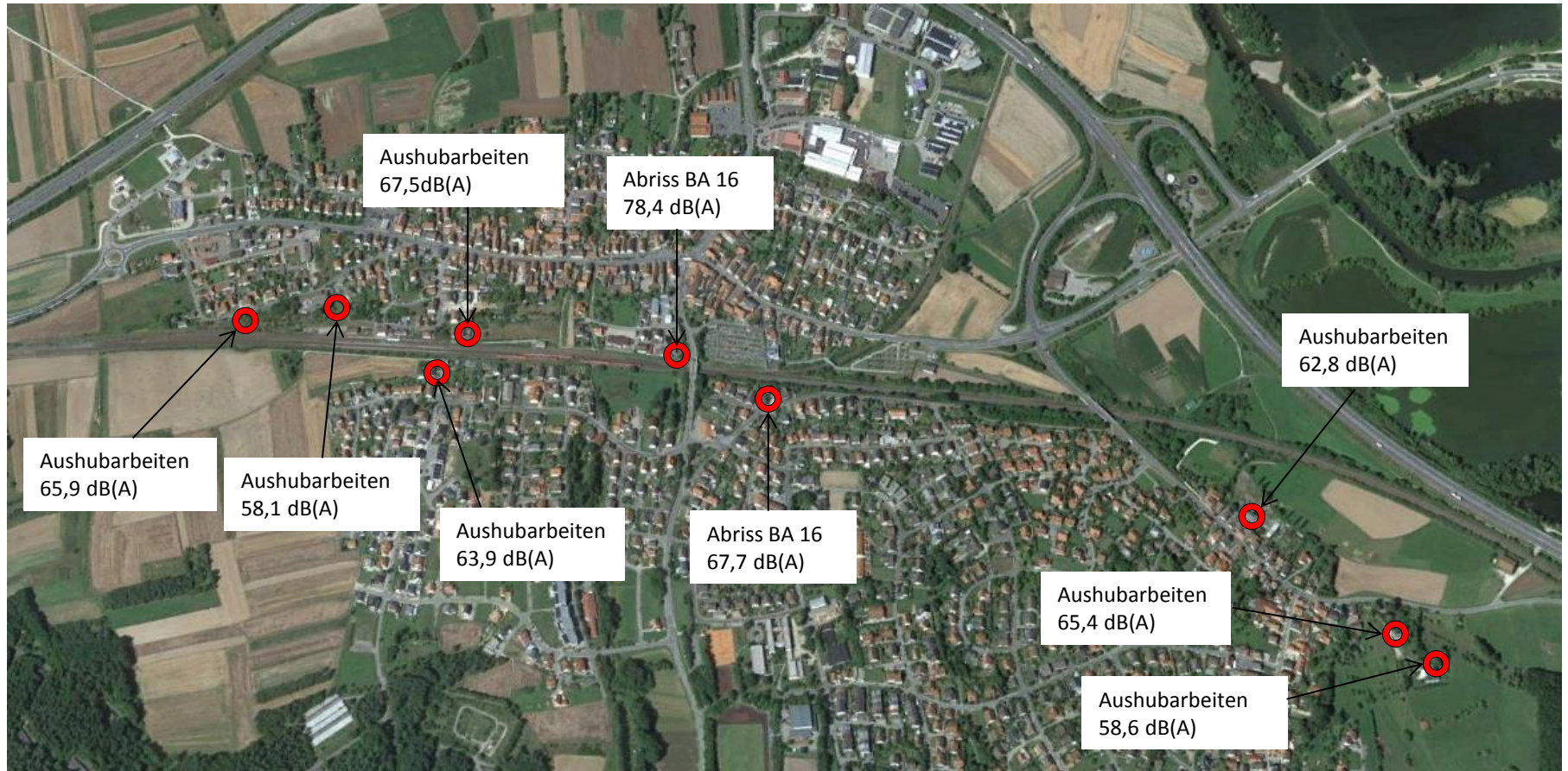
Darstellung der gemittelten Schallpegel während repräsentativen Bauarbeiten im Zeitraum 11.01.2016 bis 11.02.2016
