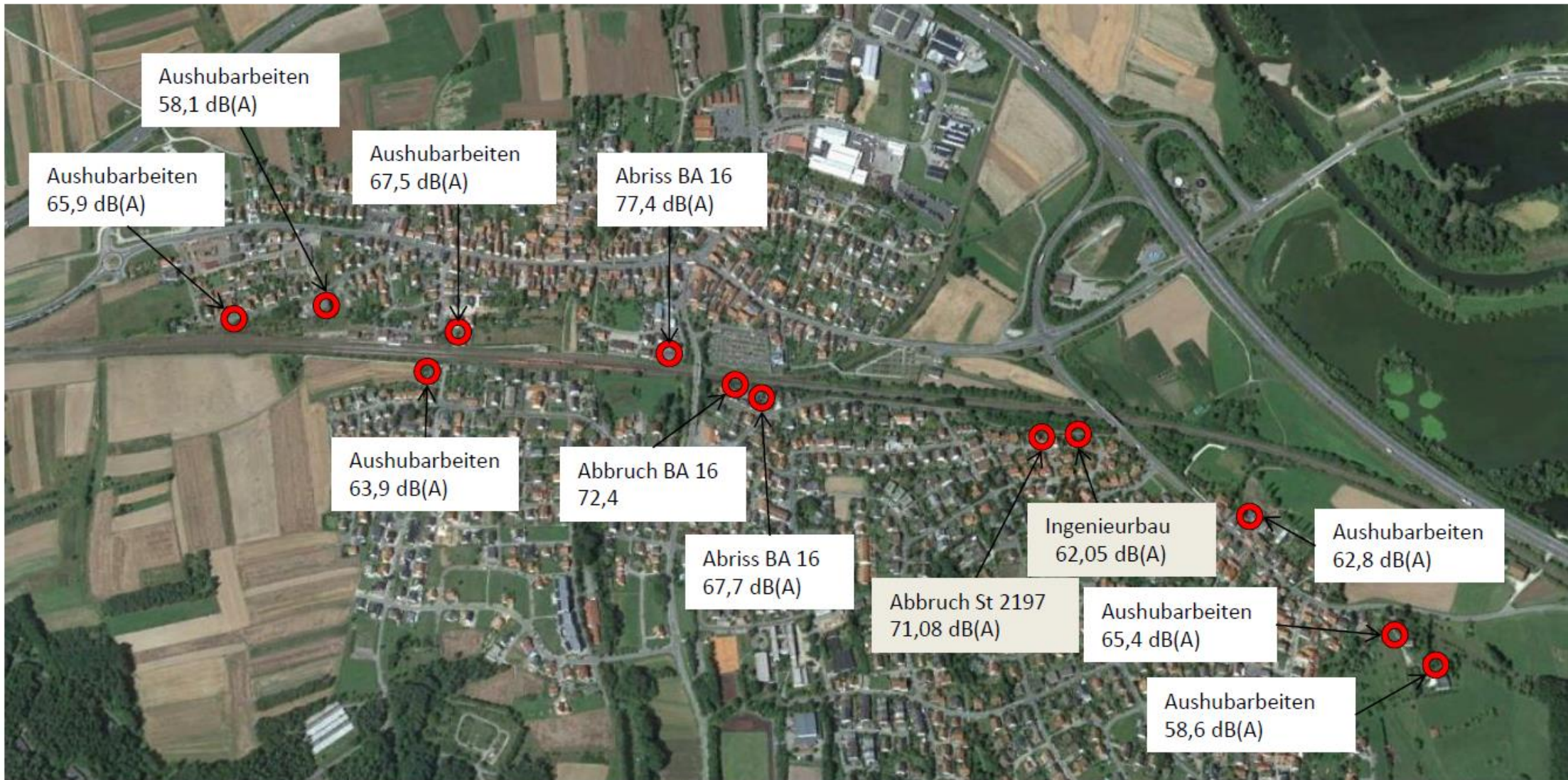
Darstellung der gemittelten Schallpegel während repräsentativen Bauarbeiten im Zeitraum 11.01.2016 bis 11.03.2016
