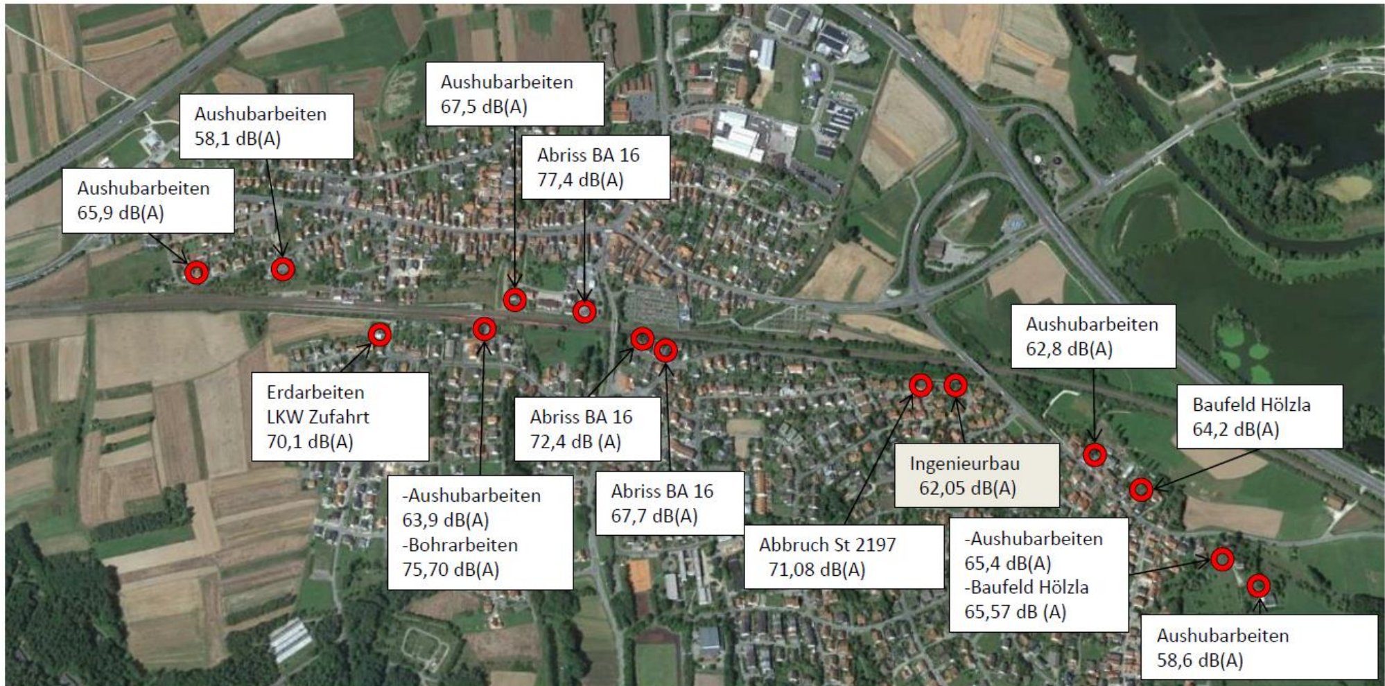
Darstellung der gemittelten Schallpegel während repräsentativen Bauarbeiten im Zeitraum 11.01.2016 bis 15.04.2016
