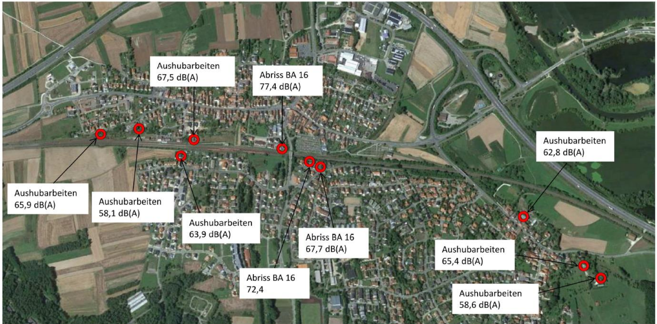
Darstellung der gemittelten Schallpegel während repräsentativen Bauarbeiten im Zeitraum 11.01.2016 bis 19.02.2016
