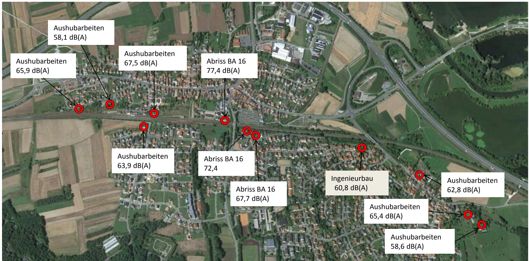
Darstellung der gemittelten Schallpegel während repräsentativen Bauarbeiten im Zeitraum 11.01.2016 bis 26.02.2016
